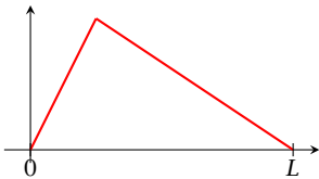
FIGURA 1: Condició inicial no diferenciable però perfectament admissible des d'un punt de vista físic.
