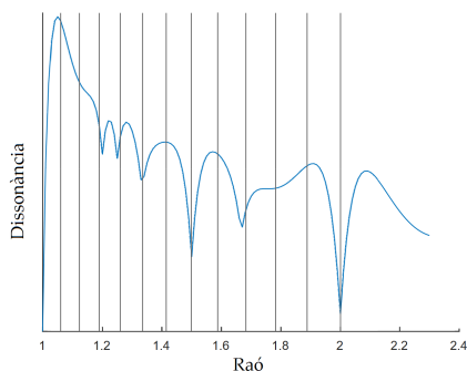
FIGURA 10: Disposició de les notes de l'escala temperada a la gràfica de dissonància.
